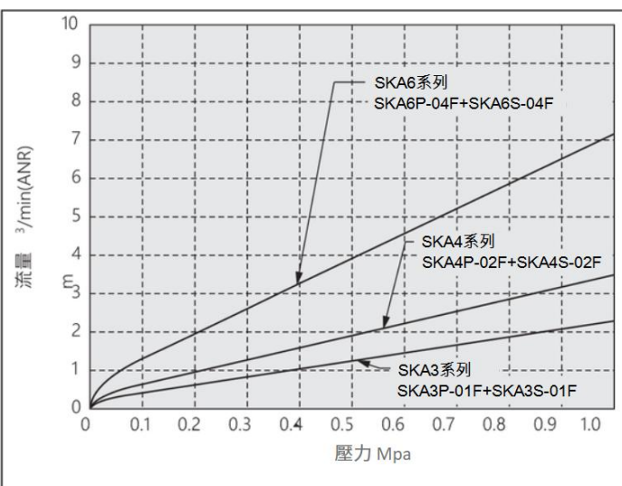
壓力損失 - 空氣 雙邊帶單向閥
