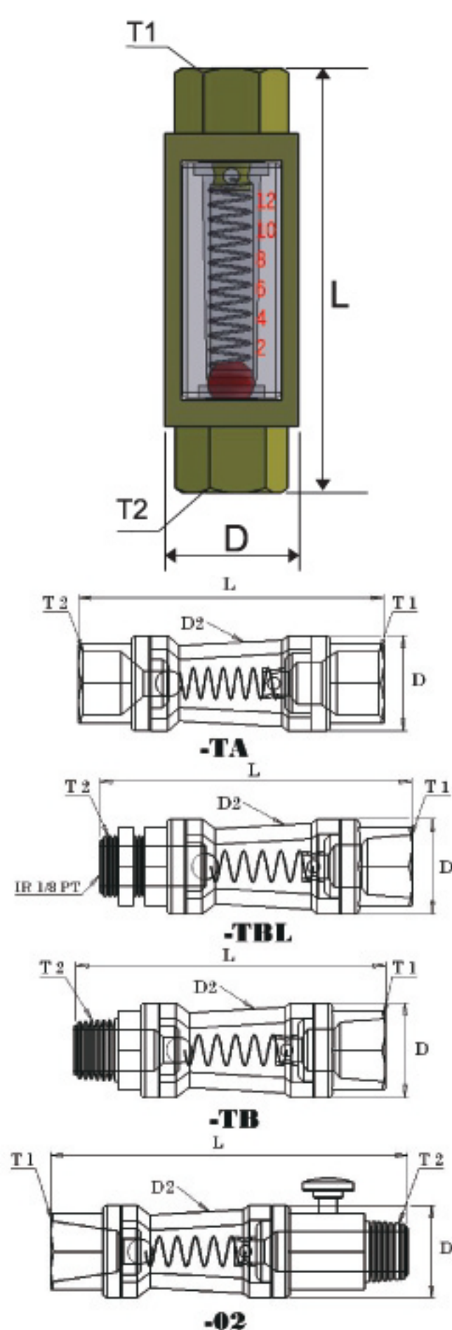
▲ SK-01TBL 雙內牙(附螺母)
